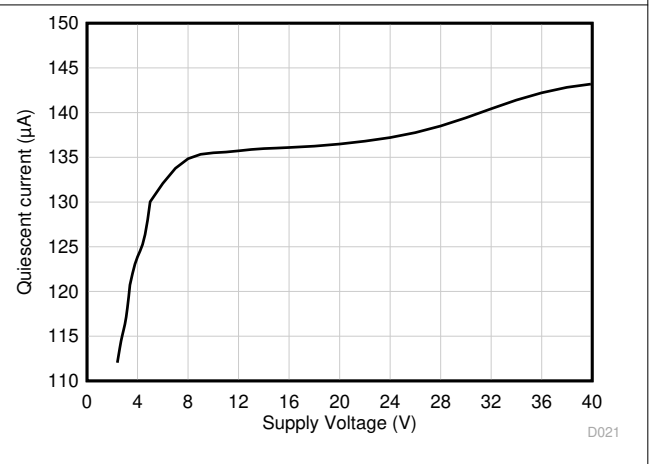
图 6-22. 静态电流与电源电压间的关系
