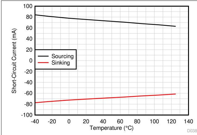
图 6-37. 短路电流与温度间的关系
