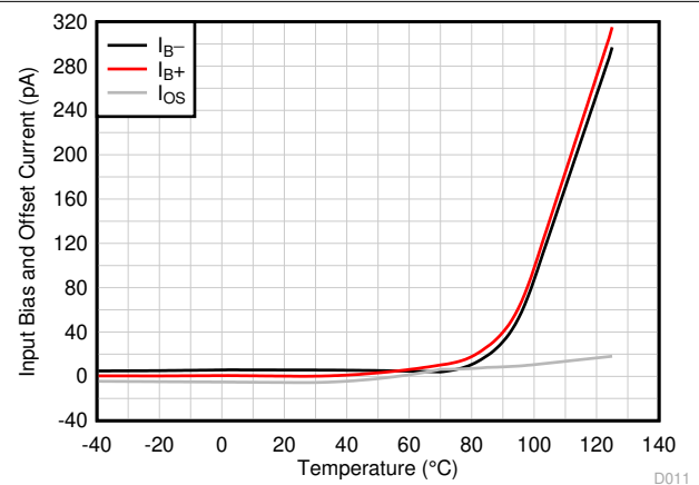
图 6-10. 输入偏置电流与温度间的关系
