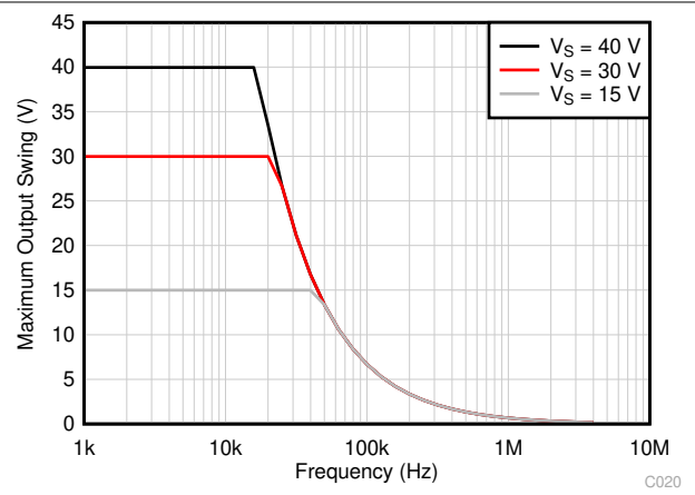
图 6-38. 最大输出电压与频率间的关系
