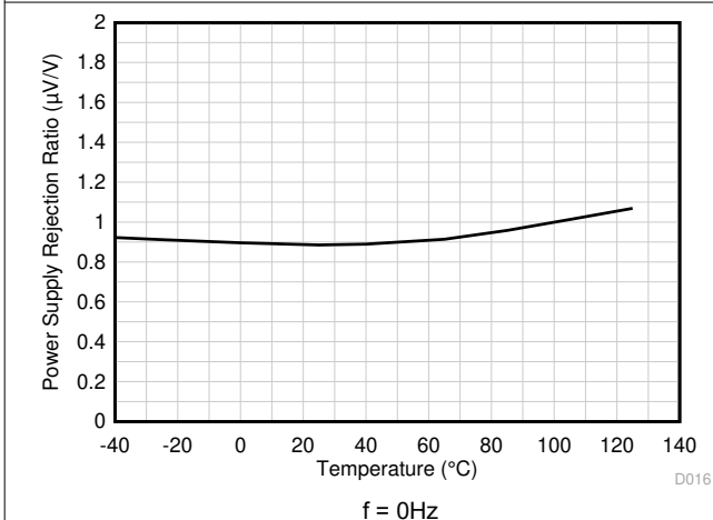
图 6-17. PSRR 与温度间的关系 (dB)
