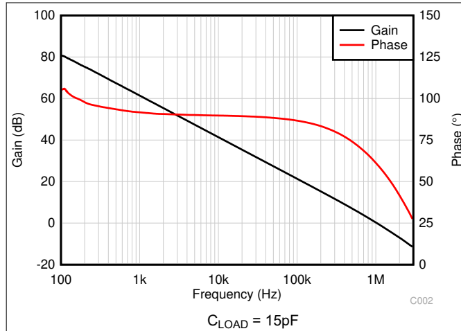
图 6-7. 开环增益和相位与频率间的关系
