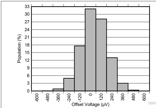
T_A = 25^\circ\text{C} 时 15462 个放大器的分配
