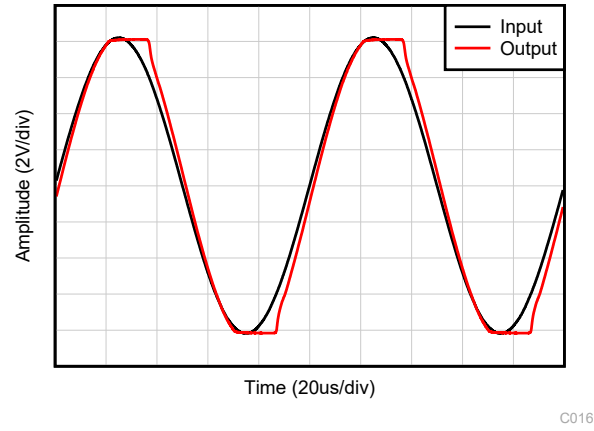
图 6-7. 无相位反转
