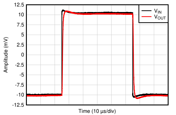
图 6-32. 无相位反转
