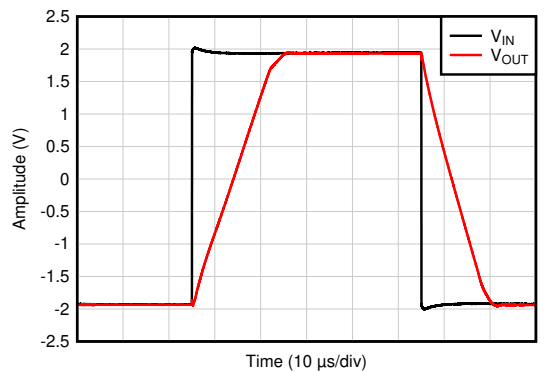
图 6-33. 过载恢复
