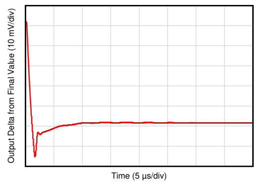
图 6-34. 小信号阶跃响应
