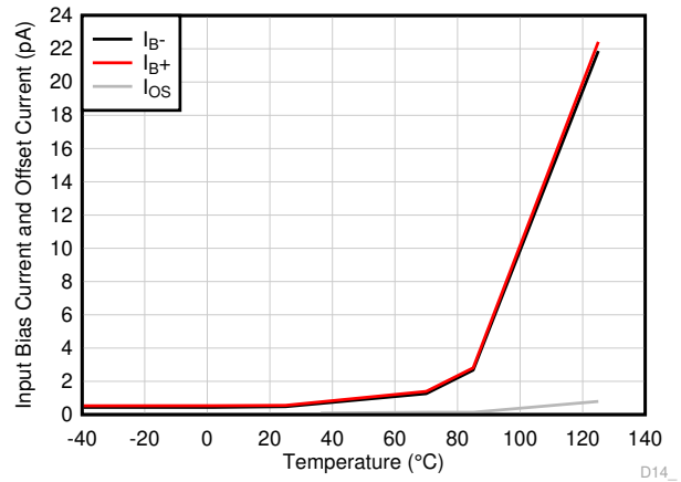
图 6-8. I_B 和 I_{OS} 与温度间的关系
