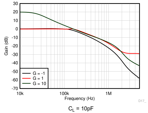
图 6-14. 闭环增益与频率间的关系
