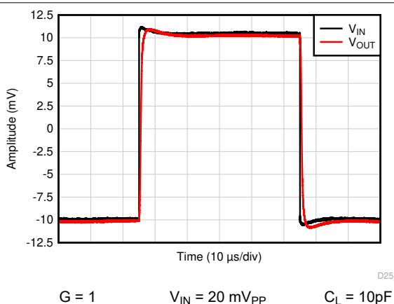
图 6-34. 小信号阶跃响应
