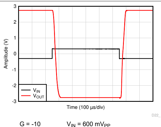
图 6-33. 过载恢复
