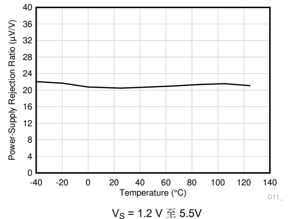
图 6-18. 直流 PSRR 与温度间的关系
