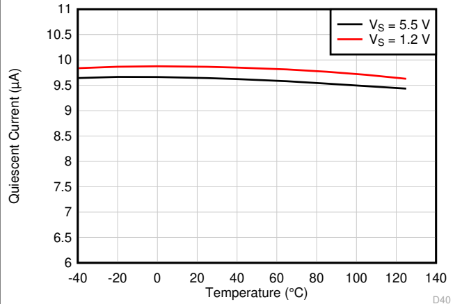
图 6-28. 静态电流与温度间的关系
