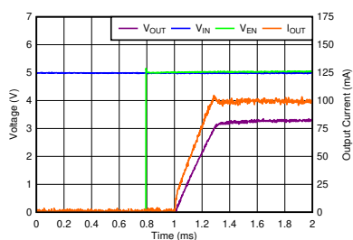
启动波形
