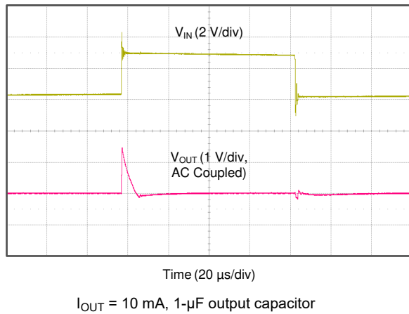
图 6-11. Line Transient
