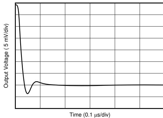
图 7-32. 大信号阶跃响应
