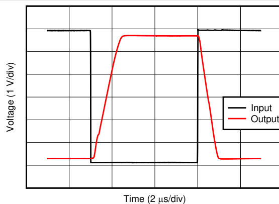
图 7-30. 过载恢复
