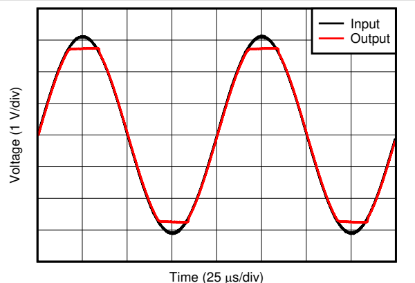
图 7-29. 无相位反转
