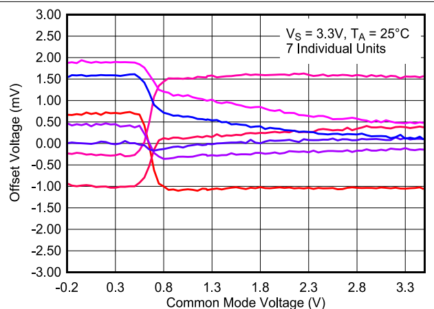
图 8-30. 失调电压与共模电压间的关系, 3.3V
