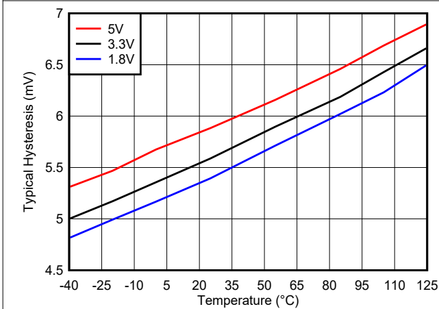
图 8-21. 迟滞电压与温度之间的关系
