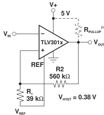
图 10-2. 添加迟滞
