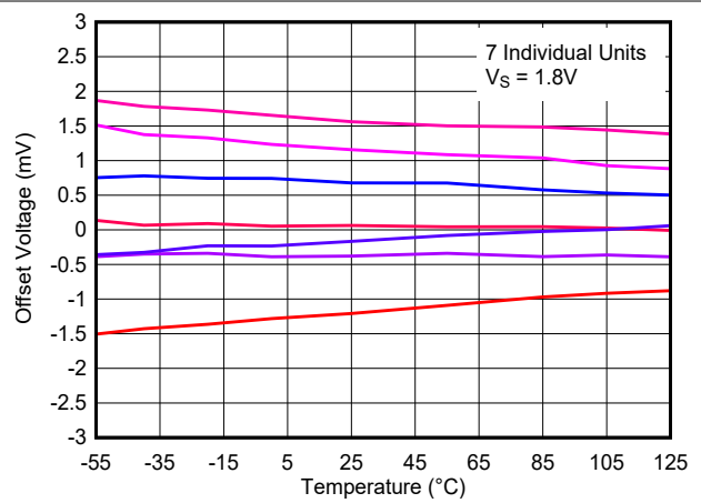
图 8-26. 失调电压与温度间的关系, 1.8V
