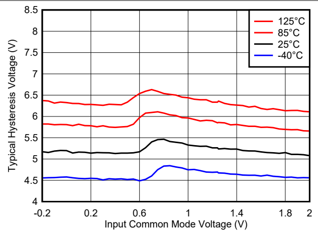
图 8-22. 迟滞电压与共模间的关系, 1.8\text{V}
