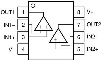
DGK、PW 封装 8 引脚 VSSOP、TSSOP 顶视图
