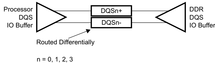
图 8-57. DQS Topology
