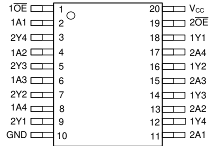
图 4-1. PW 封装，20 引脚 TSSOP (顶视图)
