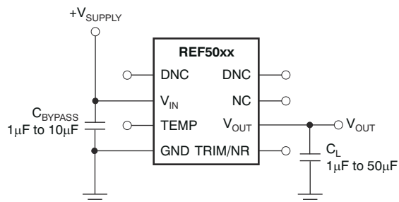
图 8-6. 基本连接
