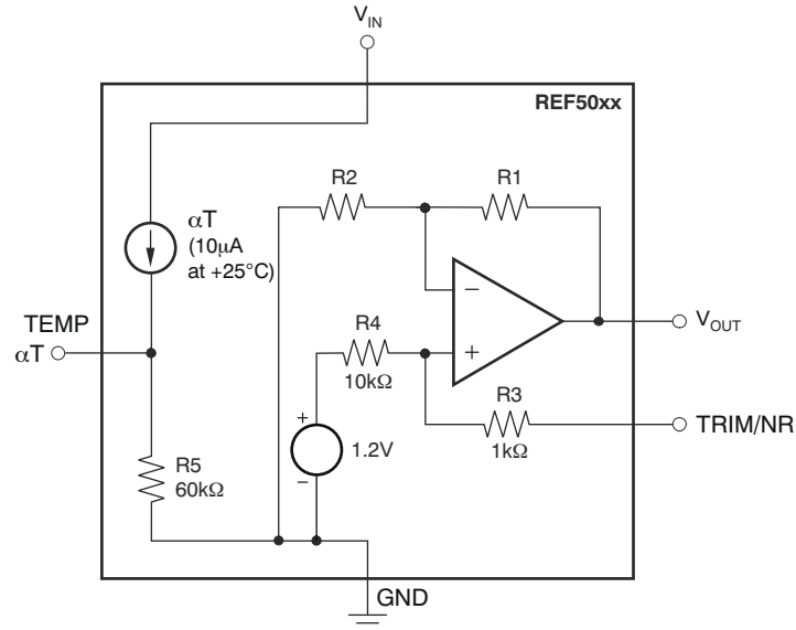
图 8-1. REF50xxI、REF50xxAI 方框图
