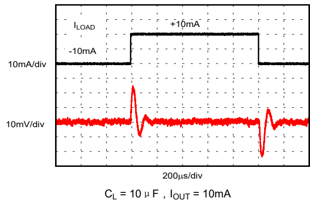
图 6-20. 负载瞬态
