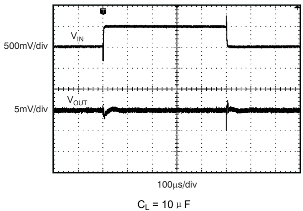
图 6-22. 线路瞬态
