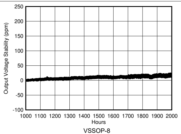
图 6-24. REF50xx 长期稳定性（后 1000 小时）
