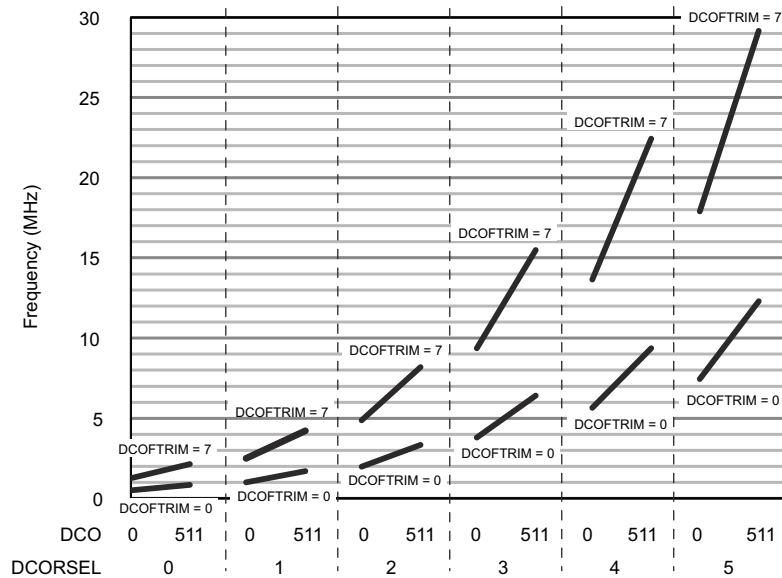
图 8-5. 典型 DCO 频率
