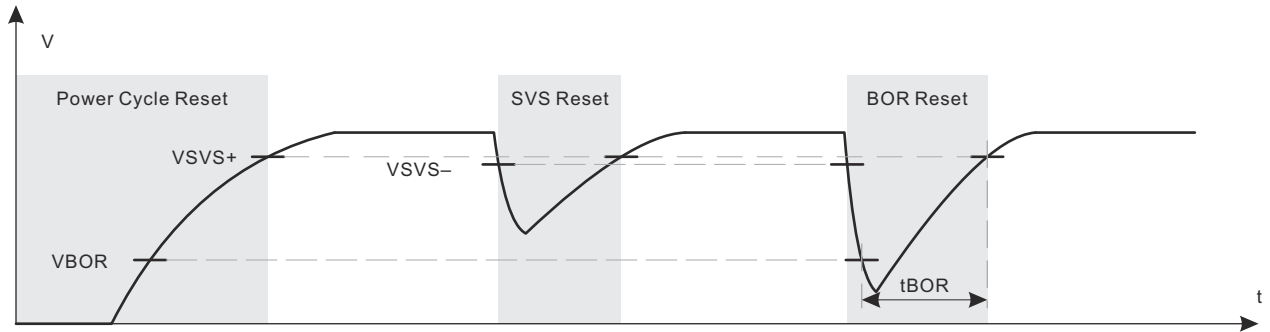
图 8-4. 重启、SVS 和 BOR 复位条件
