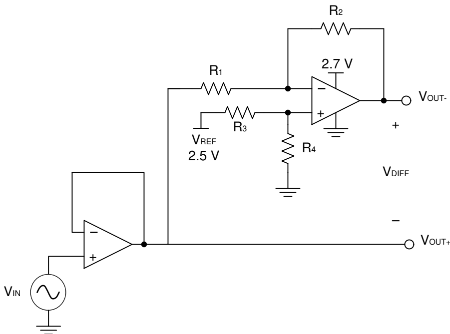
图 8-1. 单端输入转差分输出原理图
