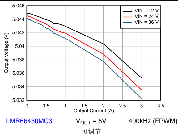
图 8-28. 线性 and 负载调整率
