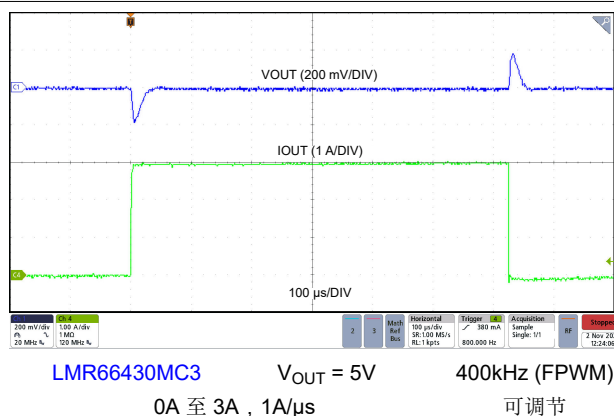
图 8-30. 负载瞬态
