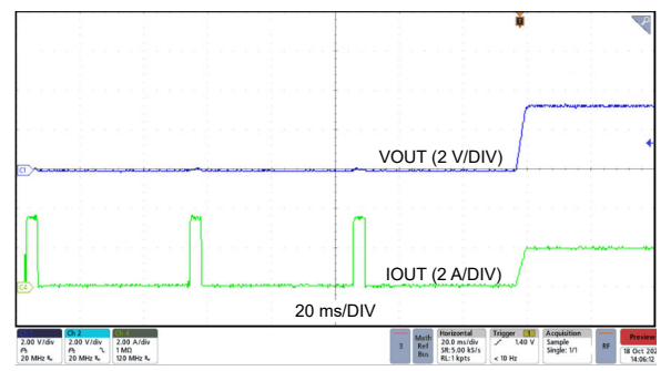
图 7-14. 退出断续
