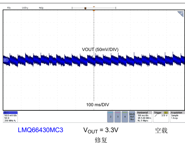
图 8-15. 输出电压纹波
