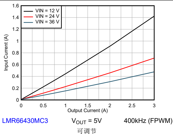
图 8-29. 输入电流与负载电流间的关系
