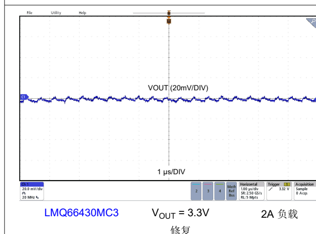
图 8-14. 输出电压纹波
