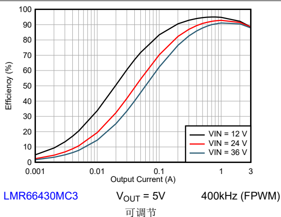
图 8-27. 效率
