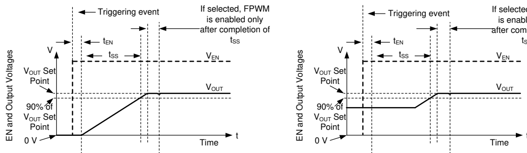
图 7-9. 带和不带预偏置电压的软启动/停止
