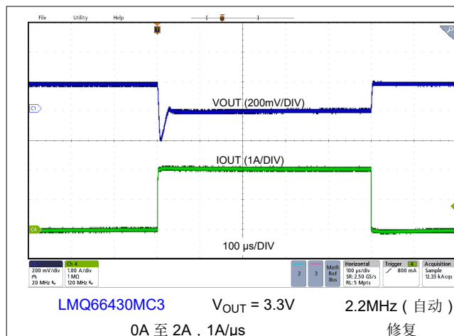
图 8-10. 负载瞬态
