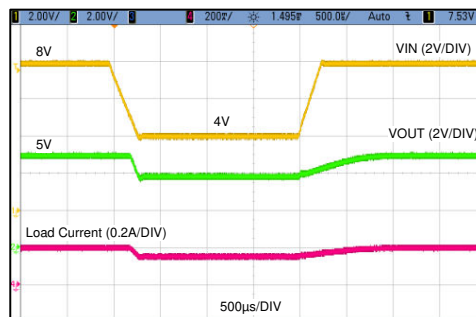
图 7-11. 典型输出从压降中恢复 (8V 至 4V)
