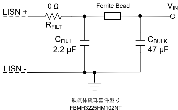
图 8-25. 典型输入 EMI 滤波器
