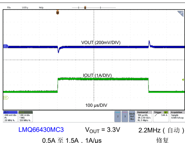
图 8-11. 负载瞬态
