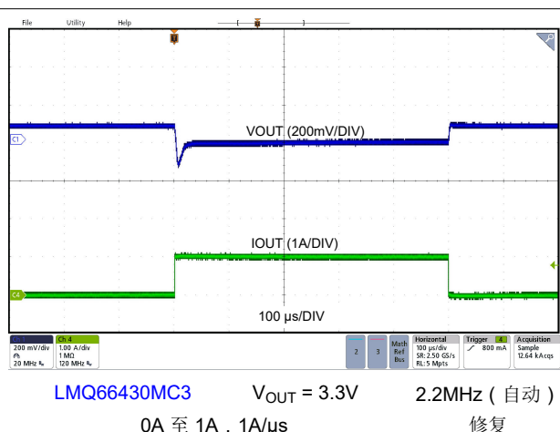
图 8-13. 负载瞬态
