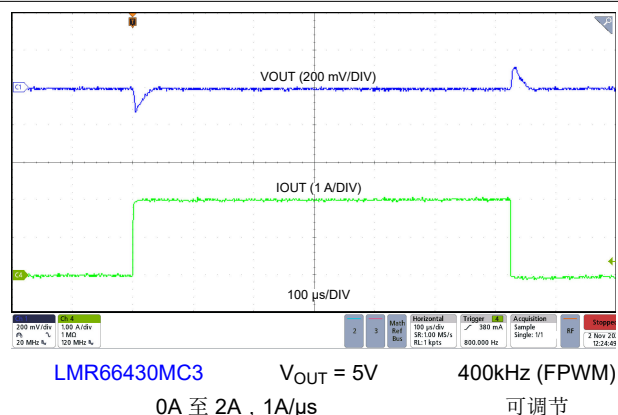
图 8-31. 负载瞬态
