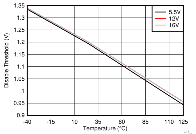
图 6-11. Disable Threshold
