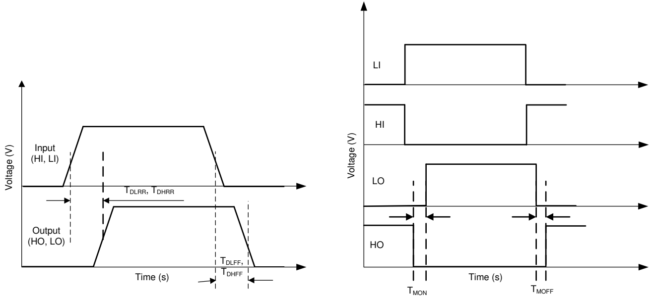
图 6-1. Timing Diagram
