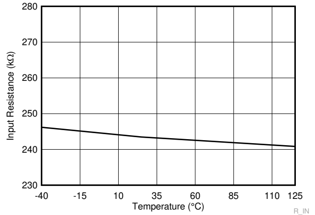
图 6-9. Input Pull-down Resistor
