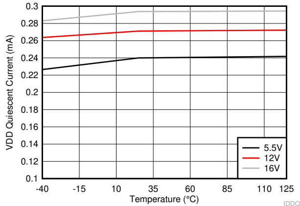
图 6-2. VDD Quiescent Current
