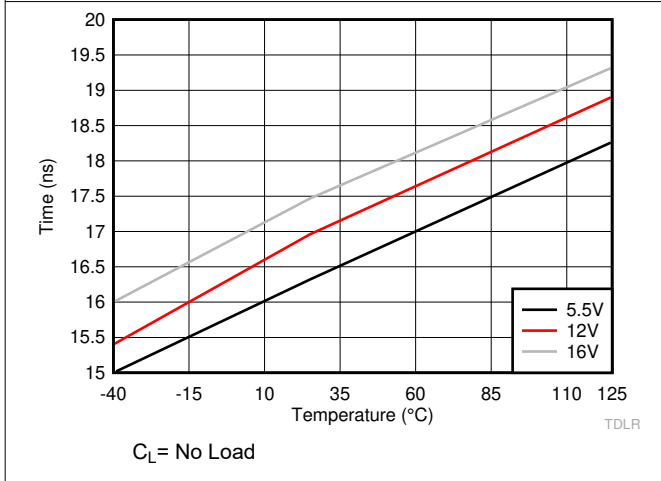
图 6-22. LO Rising Propagation Delay (TDLRR)
