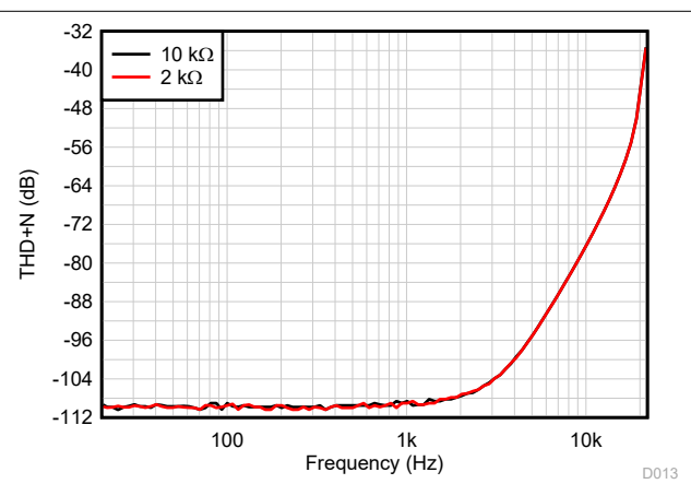
G = 1 , f = 1\text{kHz} , BW = 80\text{kHz} , V_{OUT} = 10\text{V}_{PP} , R_L 连接到 V_- 图 6-18. THD+N 比与频率间的关系, G = 1
