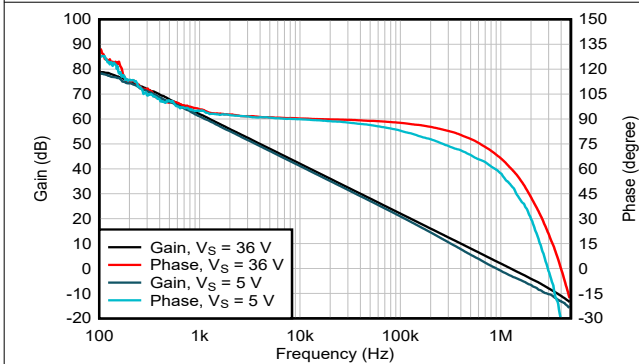
图 5-5. 开环增益和相位与频率间的关系
