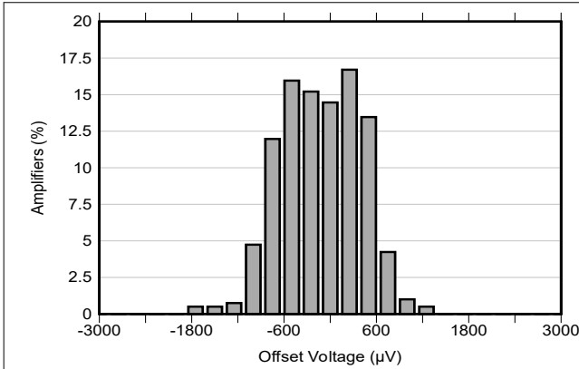
图 5-1. 失调电压产生分布
