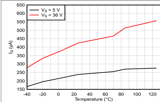
图 5-19. 静态电流与温度间的关系
