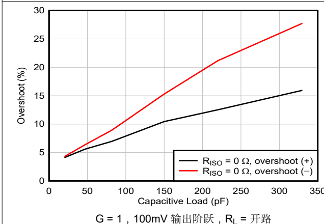
图 5-21. 小信号过冲与容性负载间的关系
