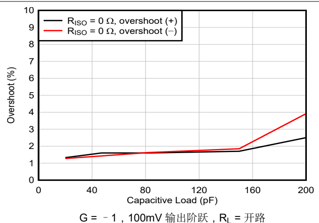
图 5-22. 小信号过冲与容性负载间的关系
