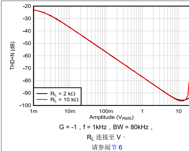
图 5-17. THD+N 与输出振幅间的关系, G = -1
