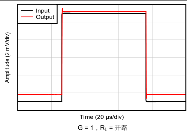
图 5-24. 过载恢复 (正轨)
