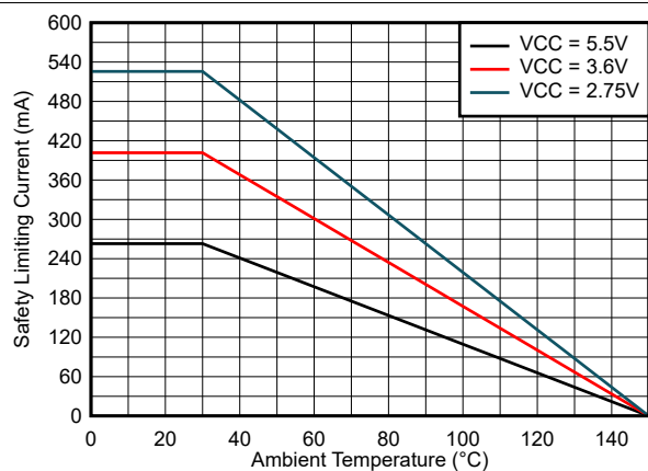
图 5-1. 宽体 SOIC (DW-16) 封装安全限制电流的热降额曲线
