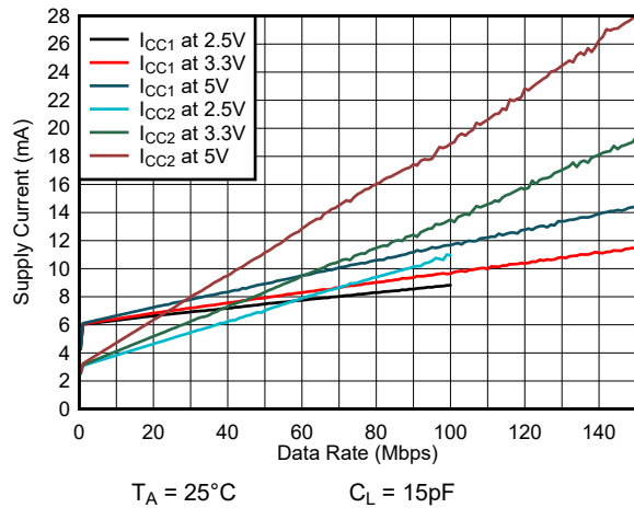
图 5-3. ISO6441 或 ISO6441F 电源电流与数据速率间的关系 (15pF 负载)
