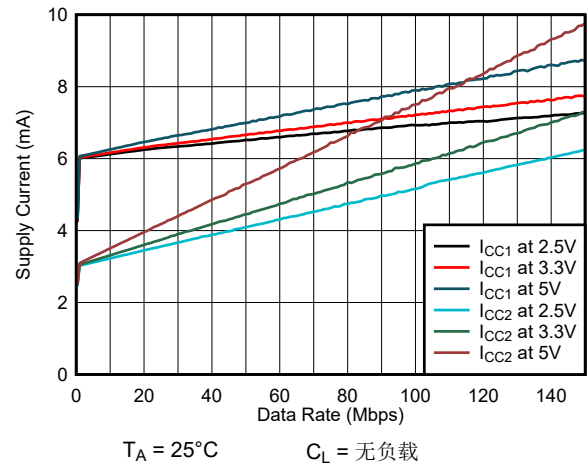
图 5-4. ISO6441 或 ISO6441F 电源电流与数据速率间的关系 (无负载)
