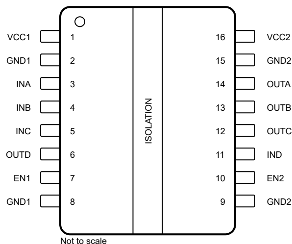
图 4-1. ISO6441 和 ISO6441F 顶视图
