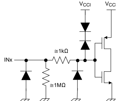
图 7-4. 输入 (INx) 默认低电平 (带 F 后缀的器件) 原理图
