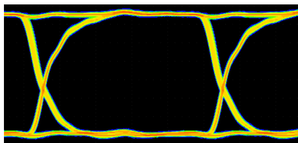
图 8-4. 100Mbps PRBS 2 16 - 1、3.3V 和 25°C 下的 ISO644x 眼图
