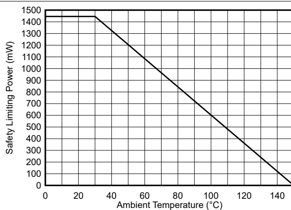
图 5-2. 宽体 SOIC (DW-16) 封装安全限制功率的热降额曲线
