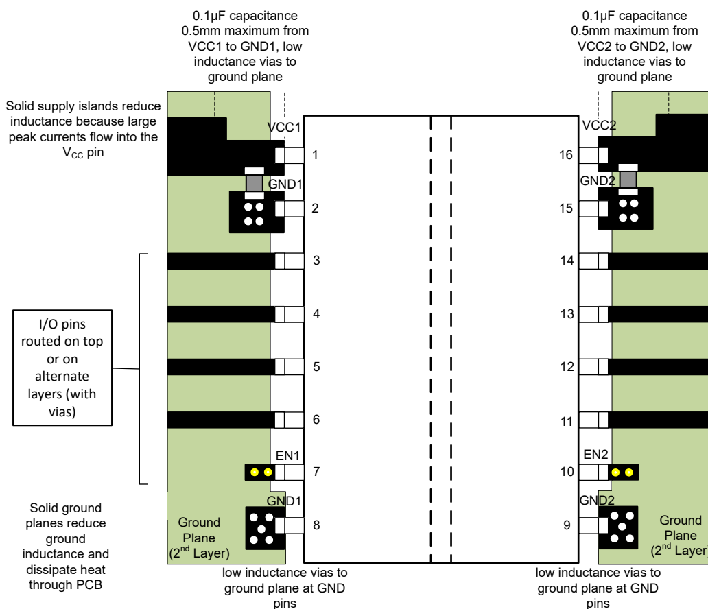
图 8-6. 布局示例
