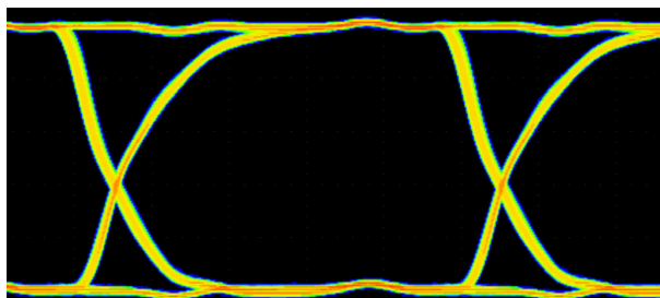
图 8-3. 100Mbps PRBS 2 16 - 1、5V 和 25°C 下的 ISO644x 眼图
