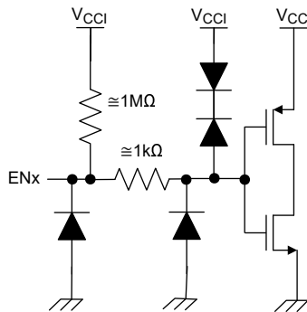
图 7-5. 使能 (ENx) 原理图
