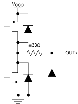
图 7-6. 输出 (OUTx) 原理图
