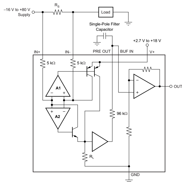
简化原理图
