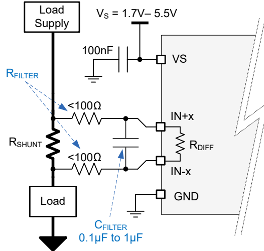
图 8-1. 输入滤波
