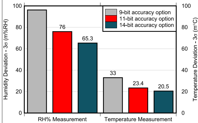
图 6-10. 平均测量灵敏度与精度选项间的关系
