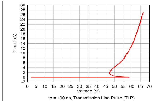
图 5-2. 负 TLP 曲线
