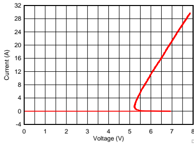
D001_Positive_TLP.grf
