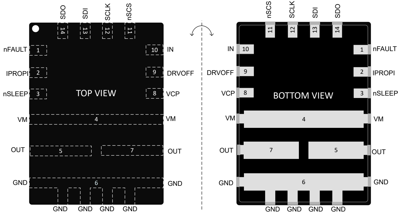
图 5-4. 采用 VQFN-HR (14) 封装的 DRV8143S-Q1 SPI 型号
