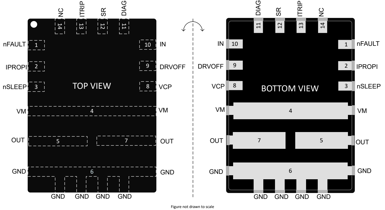
图 5-1. 采用 VQFN-HR (14) 封装的 DRV8143H-Q1 HW 型号
