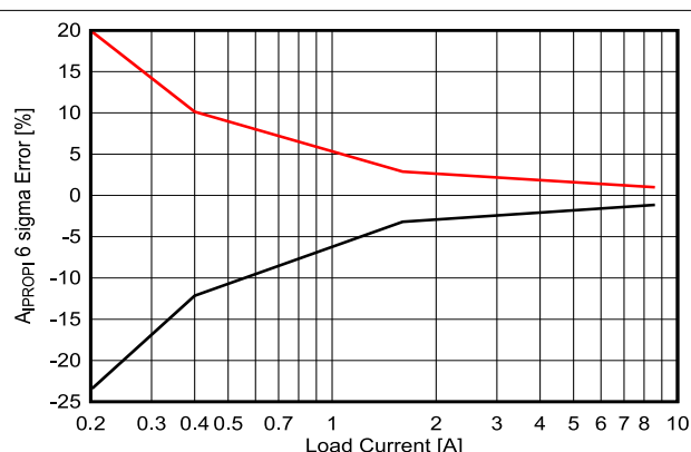
图 6-12. V_{VM} = 13.5V 时 A_{IPROPI} 增益误差与 V 负载电流之间的关系
