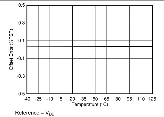
图 6-9. Offset Error vs Temperature
