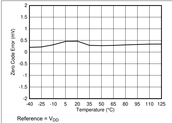
图 6-8. Zero Code Error vs Temperature
