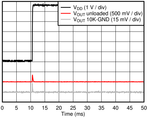
图 6-40. Power-on Glitch
