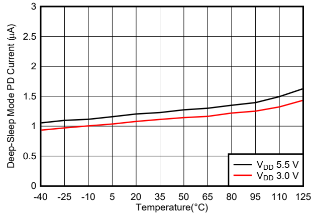
图 5-56. 断电电流与温度间的关系
