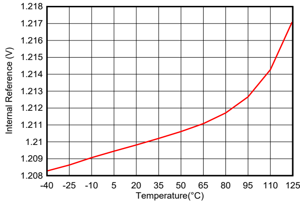
图 5-53. 内部基准与温度间的关系
