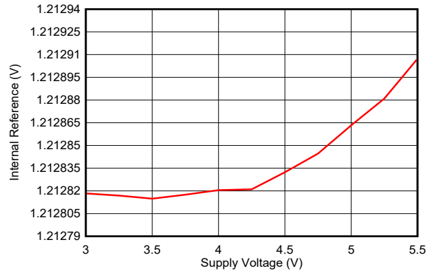
图 5-54. 内部基准与电源电压间的关系
