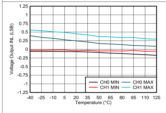
图 5-6. 电压输出 INL 与温度间的关系
