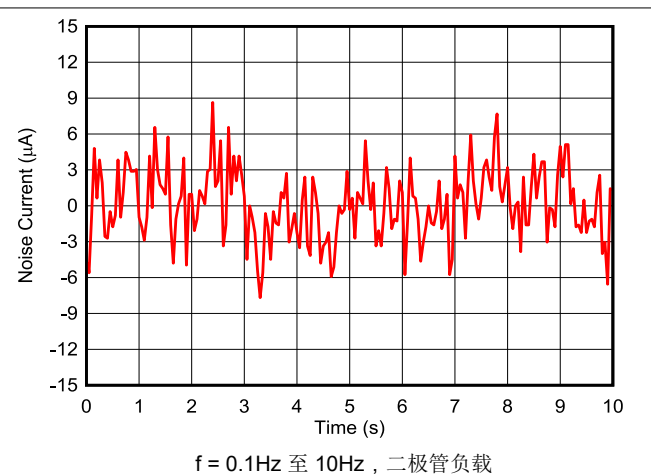
图 5-46. 电流输出闪烁噪声
