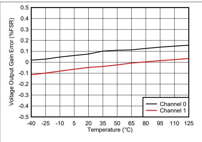
图 5-17. 电压输出增益误差与温度间的关系
