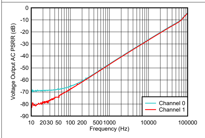
图 5-18. 电压输出交流 PSRR 与频率间的关系
