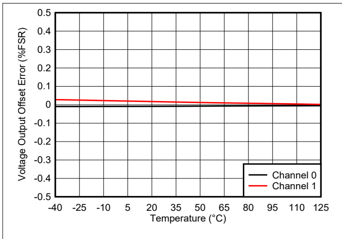
图 5-16. 电压输出偏移误差与温度间的关系
