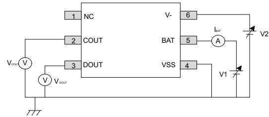
图 7-4. Test Circuit 2
