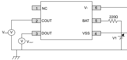
图 7-3. Test Circuit 1
