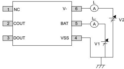
图 7-5. Test Circuit 3
