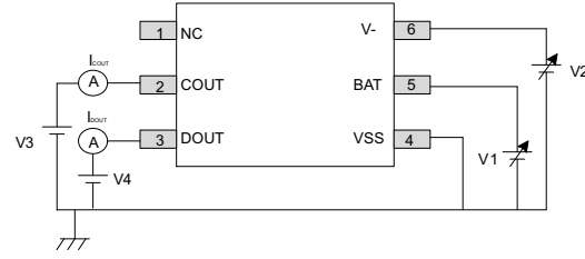
图 7-6. Test Circuit 4
