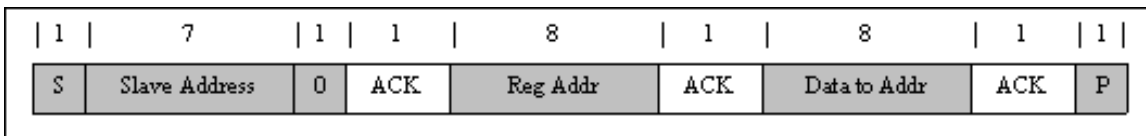
图 32. Single Write
