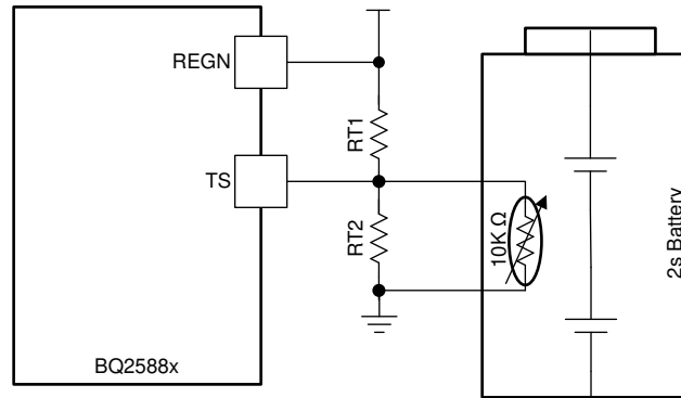
图 23. TS Resistor Network
