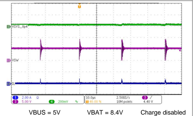
图 87. Boost Mode PFM Switching
