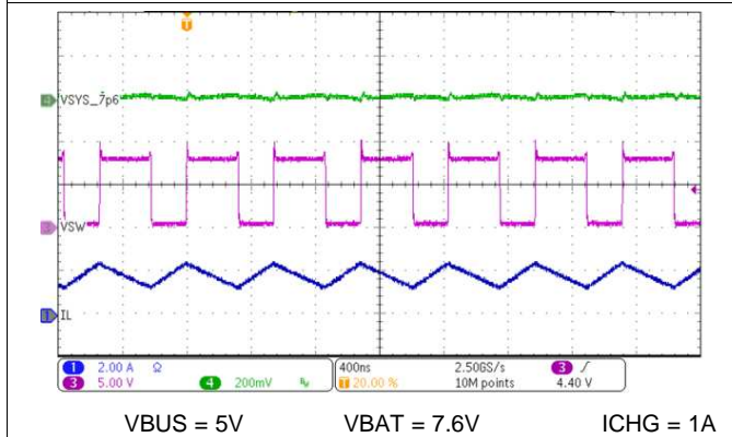
图 86. Boost Mode PWM Switching
