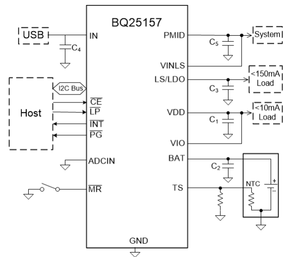
简化原理图
