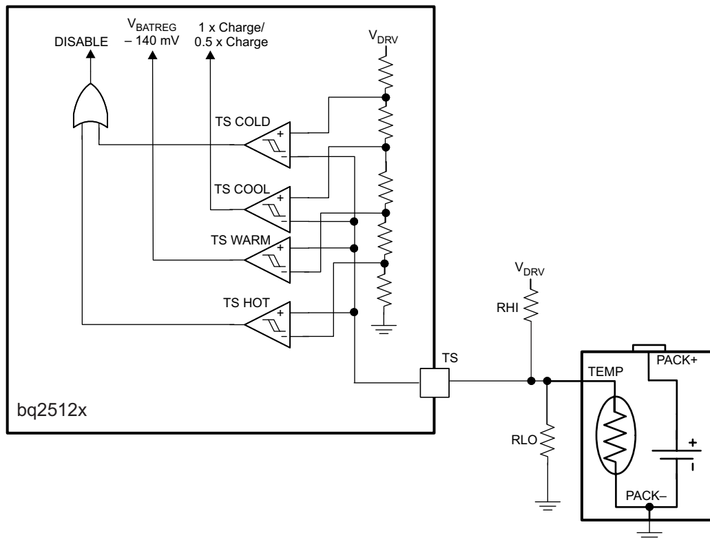
图 16. TS Circuit
