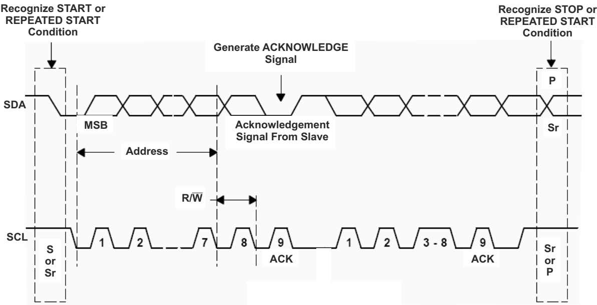
图 7-7. 总线协议
