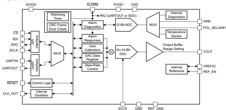
功能方框图
