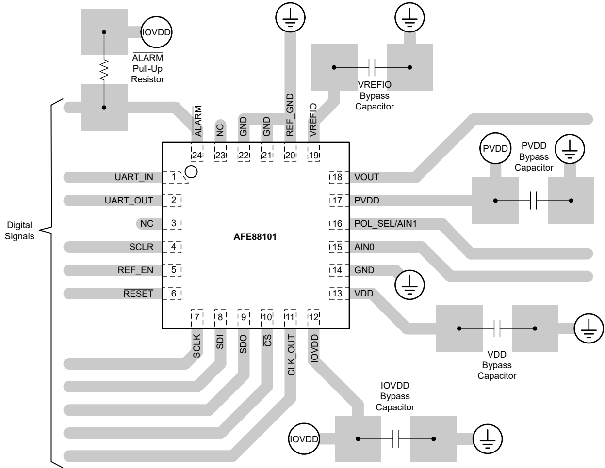
图 8-8. Layout Example
