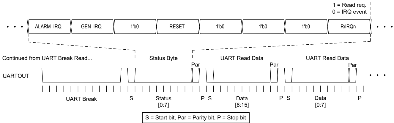
图 7-23. UARTOUT Break Data Format
