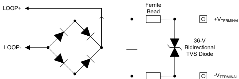
图 8-6. Loop Input Protection
