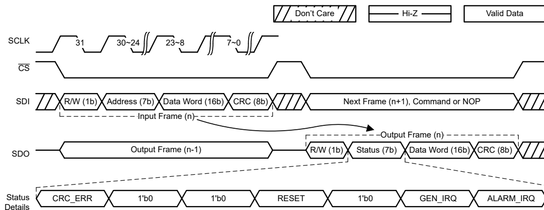
图 7-19. SPI Frame Details (Default, CRC Enabled)
