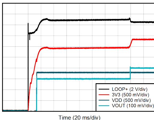
图 8-7. Circuit Start-Up
