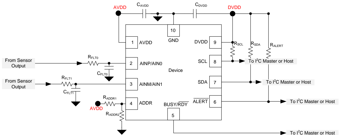
图 123. Example Circuit
