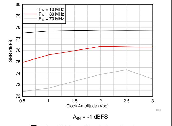
图 6-14. SNR vs Clock Amplitude
