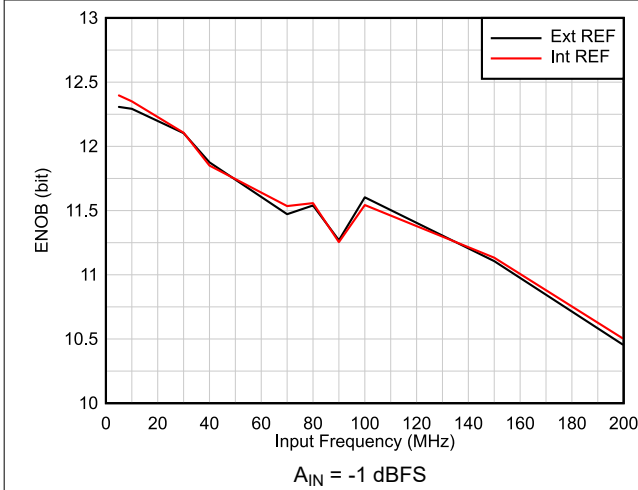
图 6-11. ENOB vs Input Frequency
