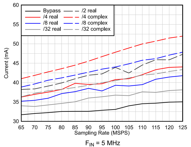
图 6-22. Current vs Decimation
