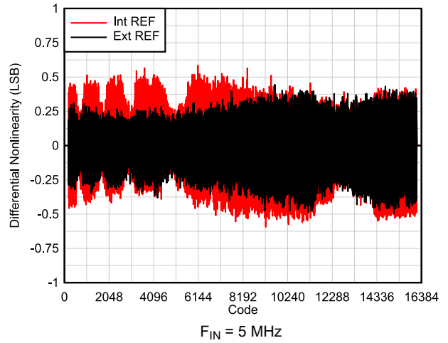
图 6-18. DNL vs Code
