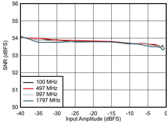
图 5-31. SNR vs Input Amplitude
