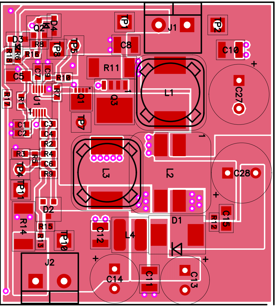
PMP2773 REV C LAYER 1-TOP
