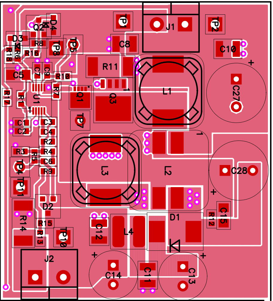
PMP2773 REV C LAYER 1-TOP
