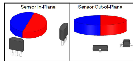
图 4. 使用一维霍尔效应传感器进行角度检测的配置
