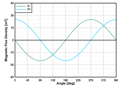
图 3. 具有 90^\circ 相移的磁场分量
