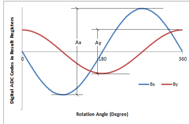
图 7. 不相等的磁场分量
