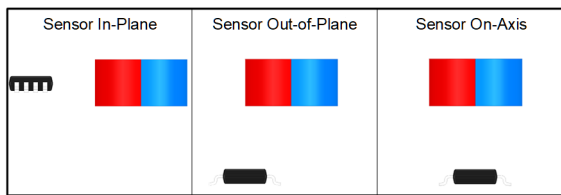
图 6. 使用多轴霍尔效应传感器进行角度检测的配置
