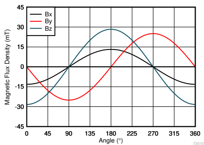
图 2. 磁通密度与磁体角度间的关系
