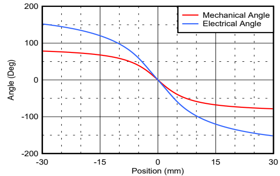
图 7. 测量角度与位置间的关系
