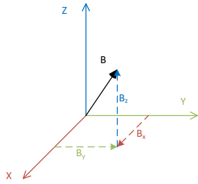
图 4. B 场矢量
