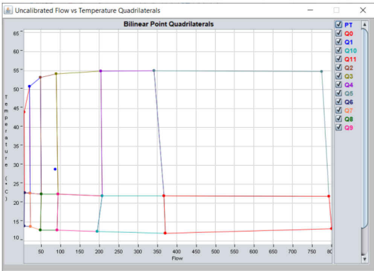
图 4-1. 校准四边形
