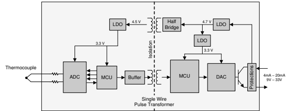
图 2. 现场发送器 - 用于数据隔离的单通道脉冲变压器
