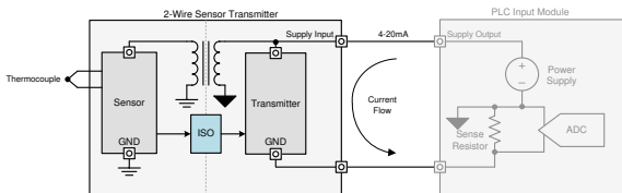
图 1. 具有 PLC 输入模块的环路供电式现场发送器
