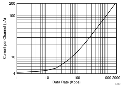
图 4. ISO7041 单通道功率与数据速率间的关系
