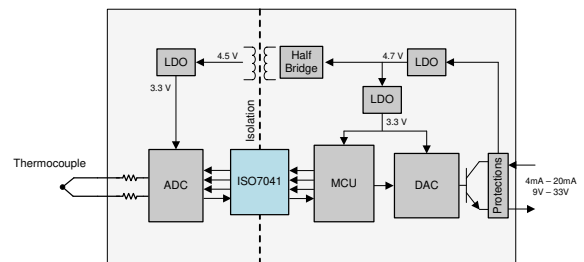
图 3. 现场发送器 - 用于多通道和双向数据隔离的 ISO7041
