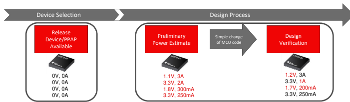
图 3. I 2 C 配置设计过程
