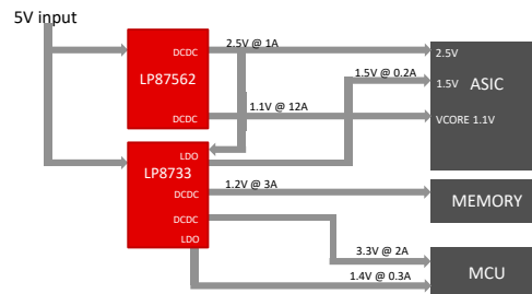
图 2. 分布式电源示例
