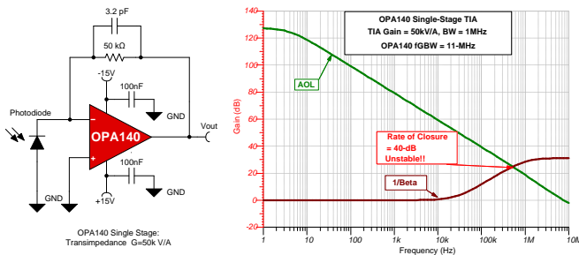
图 3. 单级 OPA140 (f GBW = 11MHz) 稳定性分析 (不稳定)
