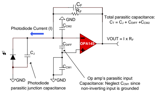
图 1. 光电二极管跨阻放大器
