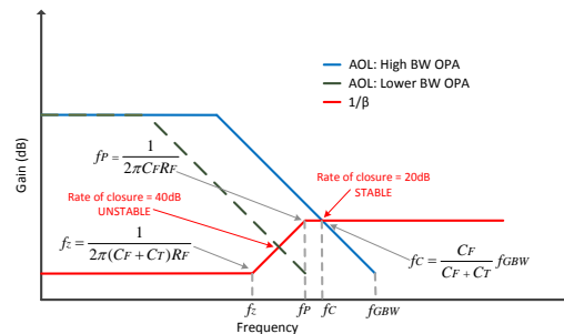
图 2. 跨阻运算放大器电路的 AOL 和 1/\beta 图
