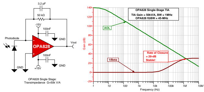
图 5. 单级 OPA828 (f GBW = 45MHz) TIA 稳定性分析 (稳定)
