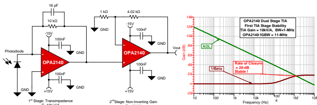
图 4. 另一种两级 OPA140 TIA 放大器 (稳定)
