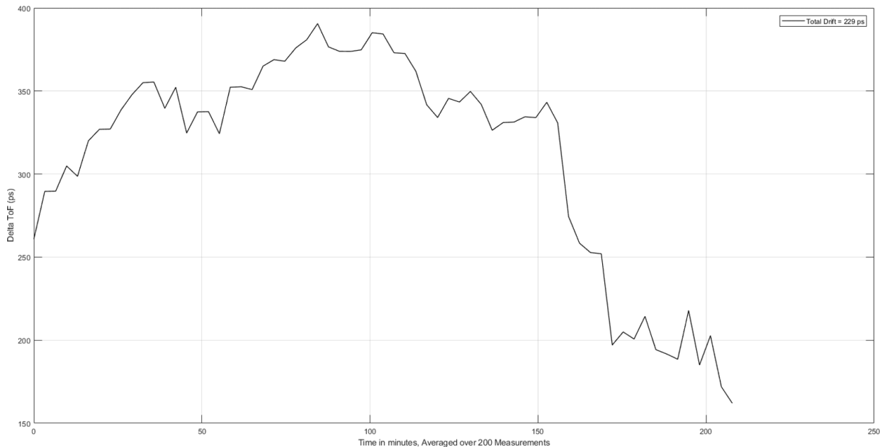
图 3. 燃气表应用的零流量漂移 (ZFD)
