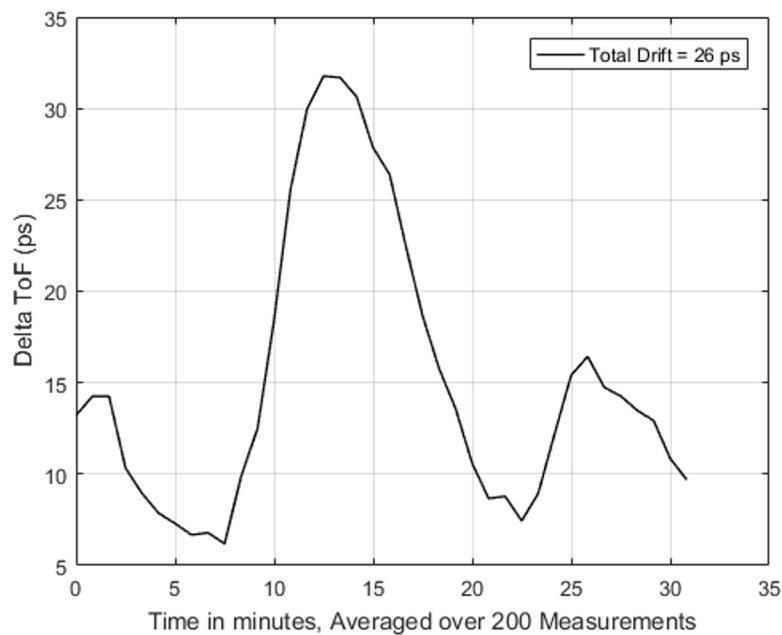
图 2. 流量计位于烘箱中时，水流量的 dTOF 零流量漂移 (ZFD)
