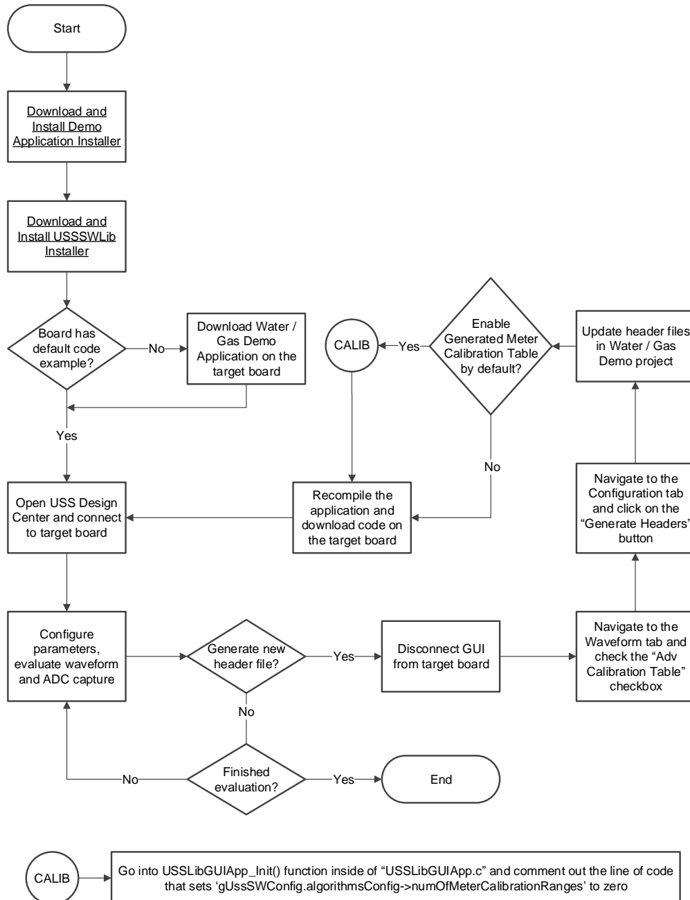
图 4. 仪表校准流程图
