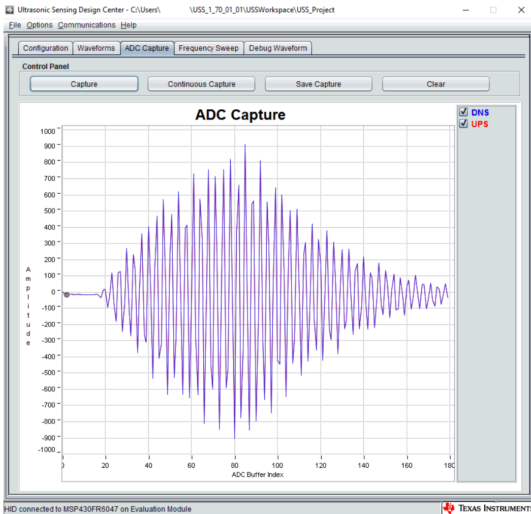
图 1. 典型的 ADC 捕获
