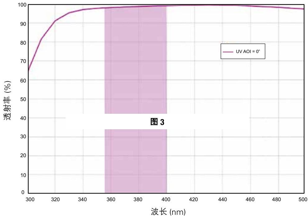
图 3: UV 光窗口 AR 涂层透射率 (最大透射区域)
