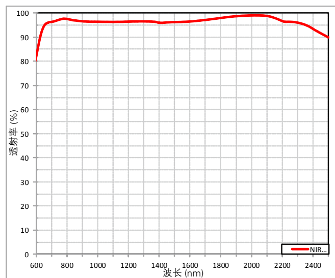
图 6: Corning Eagle XG NIR AR 涂层透射率
