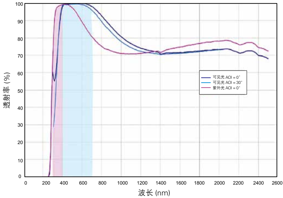
图 1: Corning 7056 可见光和紫外 (UV) 光窗口透射率响应曲线
