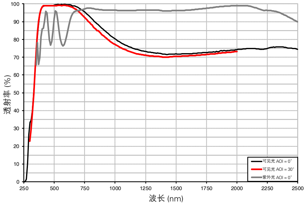
图 4: Corning Eagle XG 窗口 AR 涂层选项
