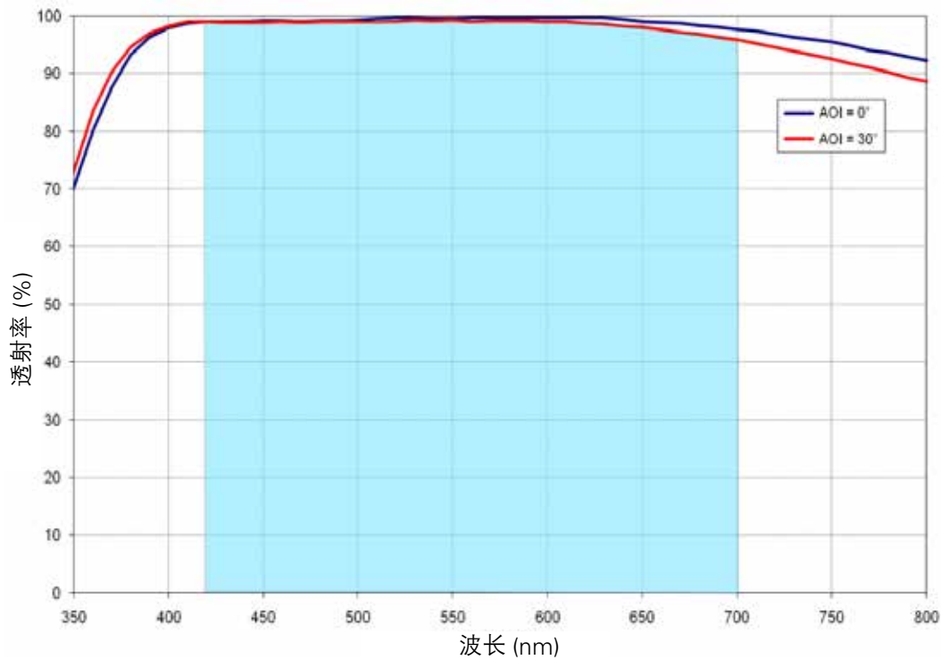
图 5: Corning Eagle XG 可见光 AR 涂层透射率
