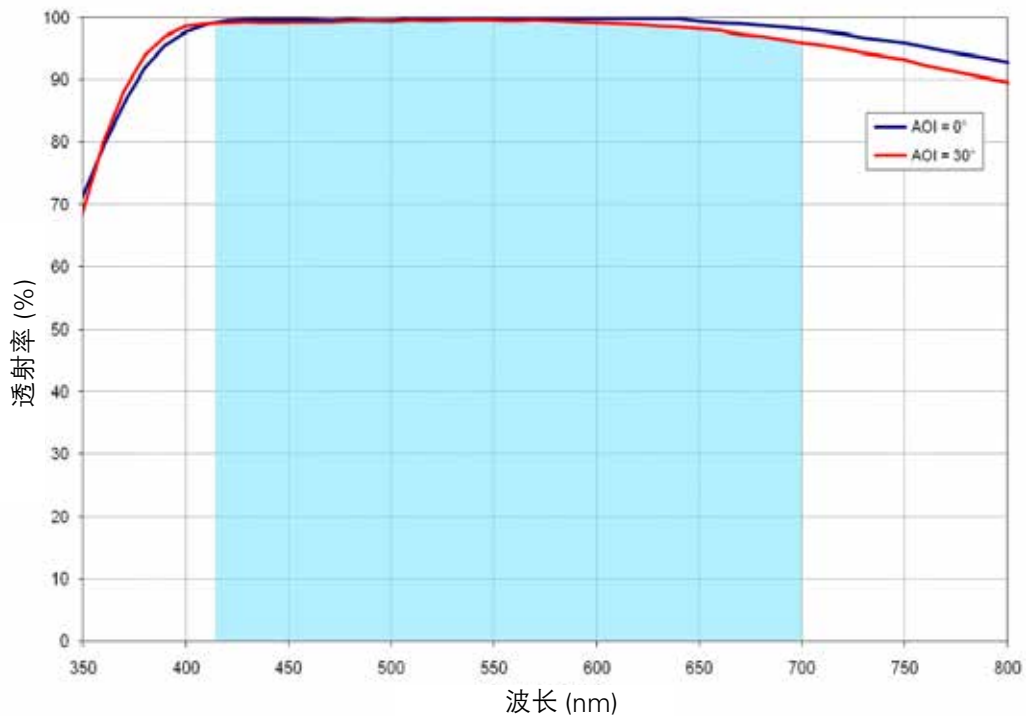
图 2: Corning 7056 可见光窗口透射率 (最大透射区域)
