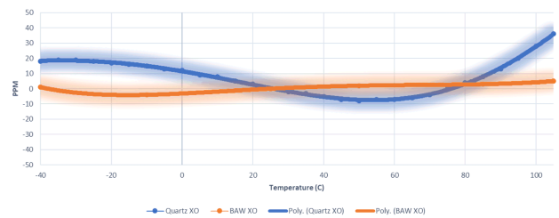
图 4. BAW 振荡器和石英的温度稳定性比较
