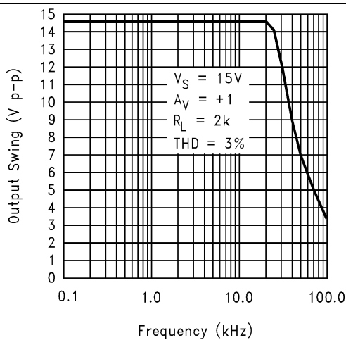
图 37. 最大输出摆幅与频率间的关系
