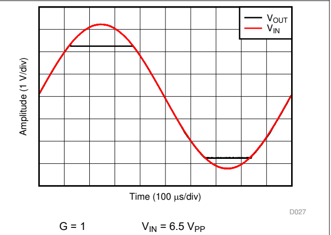
图 6-21. 无相位反转
