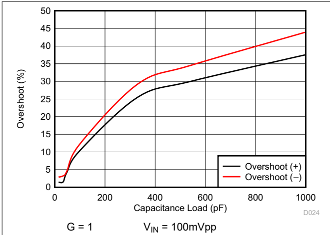
图 6-18. 小信号过冲与容性负载间的关系
