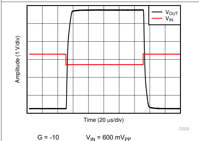
图 6-22. 过载恢复
